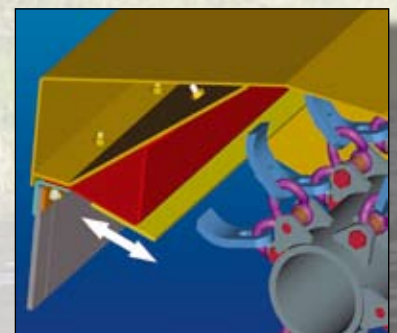
Einstellbare Häckselplatte
